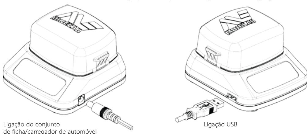
Figura 36 – Ligações USB e conjunto de ficha do BC 10
